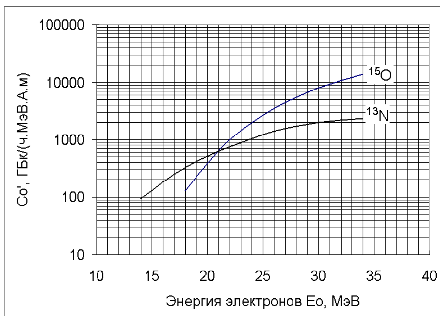
Рис.1. Зависимость постоянной скорости образования ( C_0' ) радионуклидов ^{13}\text{N} и ^{15}\text{O} от энергии электронов (вольфрамовая мишень).
